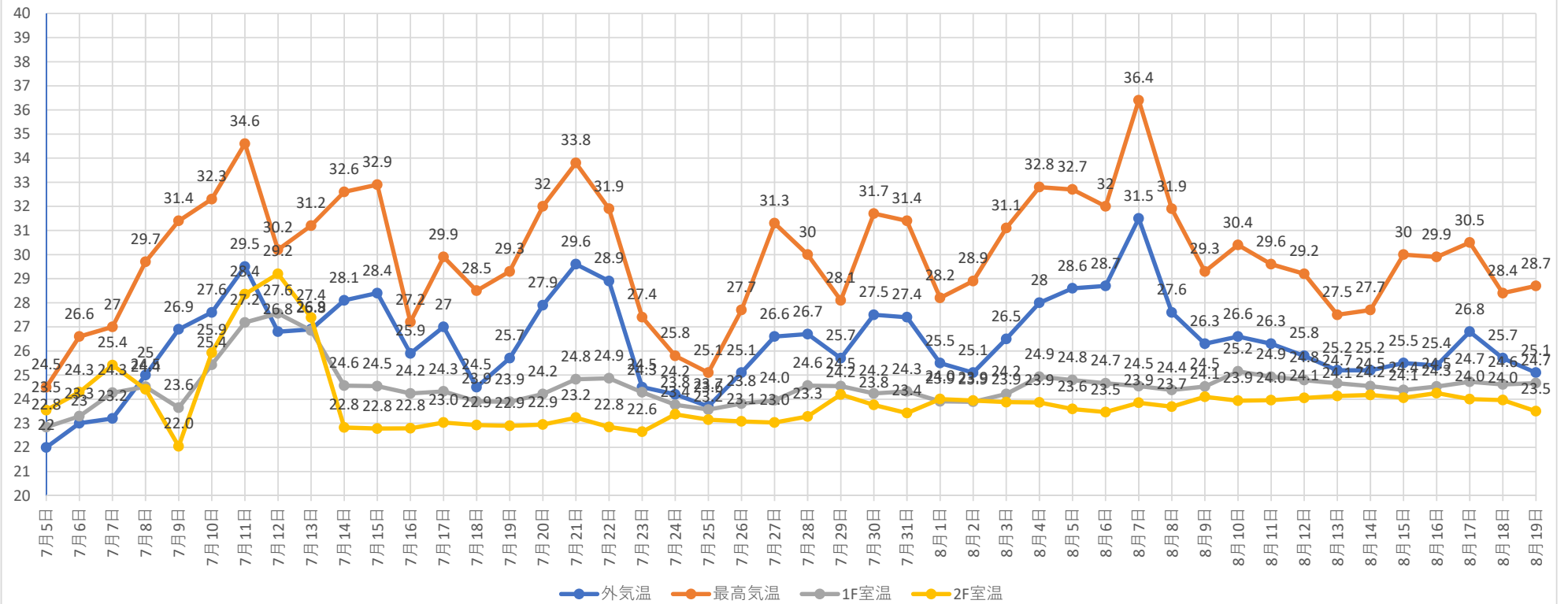
船戸山モデルハウス 温度グラフ（夏）
