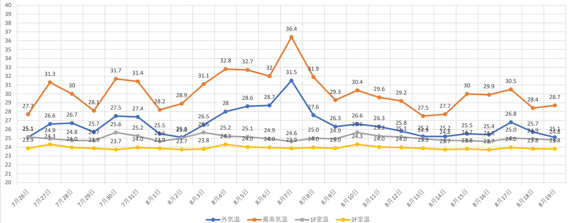
小針モデルハウス 温度グラフ（夏）
