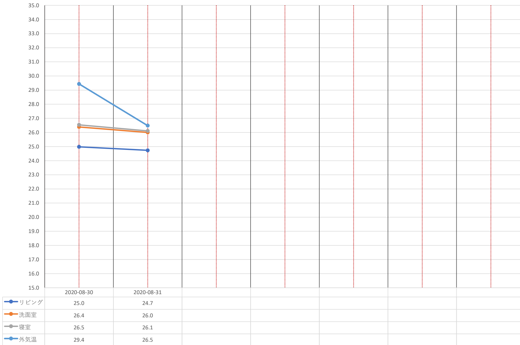
東区物見山モデルハウス 平均温度グラフ 【8/30~8/31】
