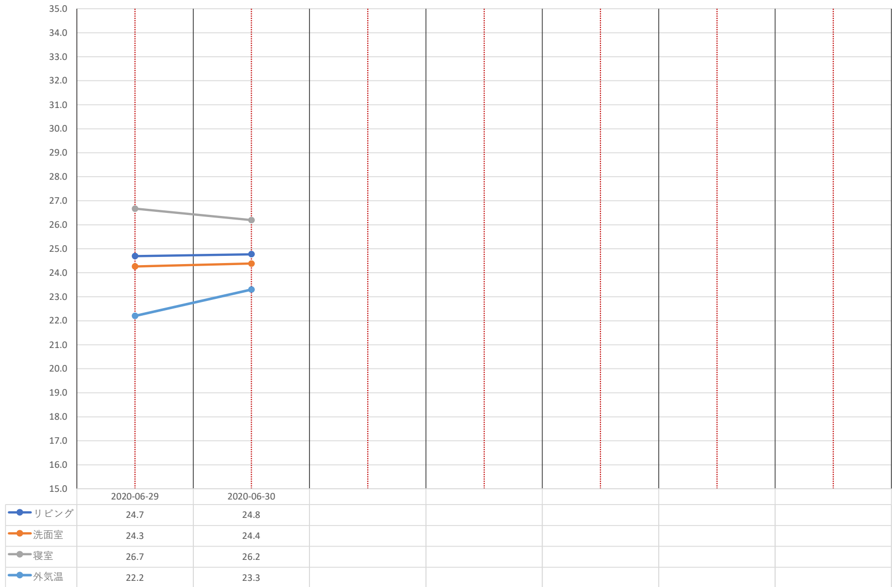
東区物見山モデルハウス 平均温度グラフ 【6/29～6/30】
