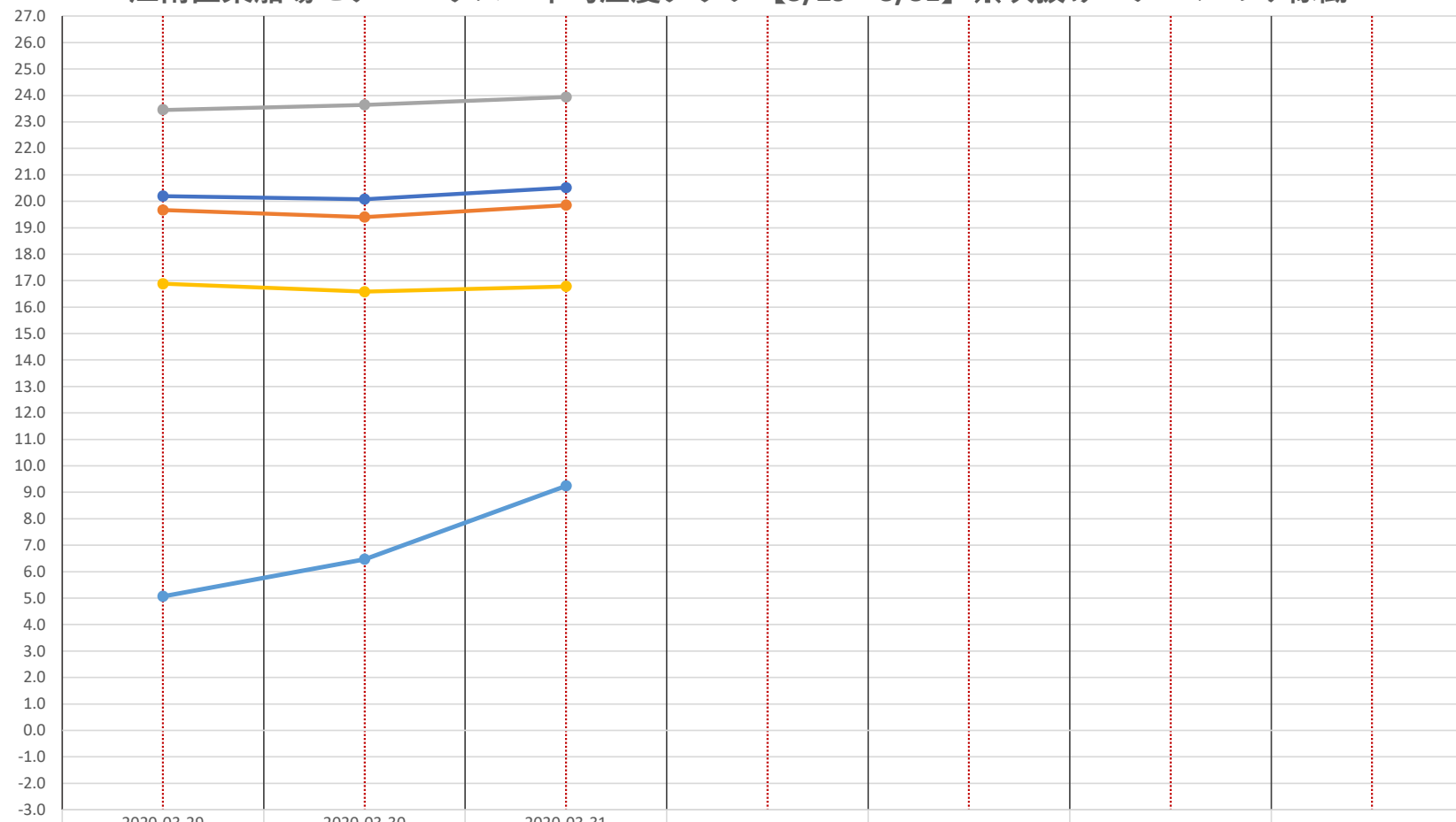
江南区東船場モデルハウス 平均温度グラフ【3/29~3/31】 ※吹抜けエアコンのみ稼働
